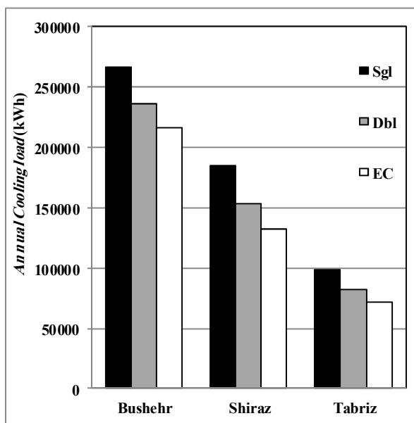
شکل (۱۲): متوسط سالانه بار سرمایش ساختمان اداری در سال برای بوشهر، شیراز و تبریز
