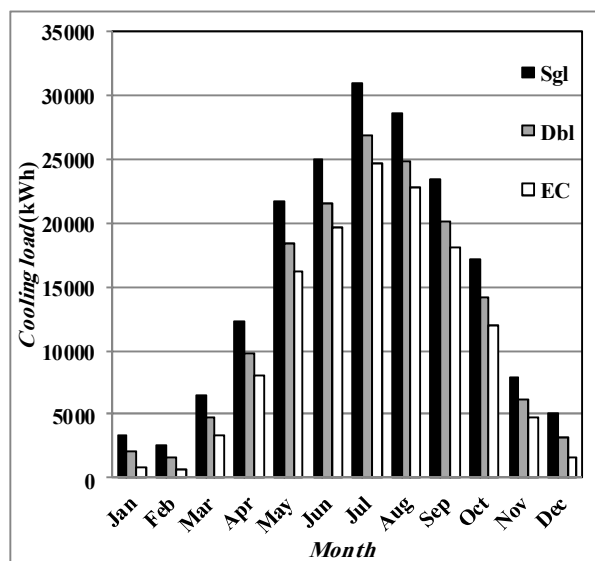
شکل (۱۰): بار سرمایش ساختمان اداری در ماه‌های سال در شیراز
