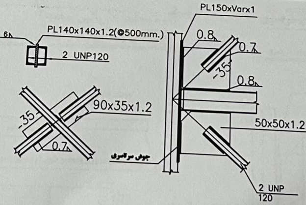
جزئیات اتصال میان دیوار و تیرچه میانبر، همگرای شتابی
