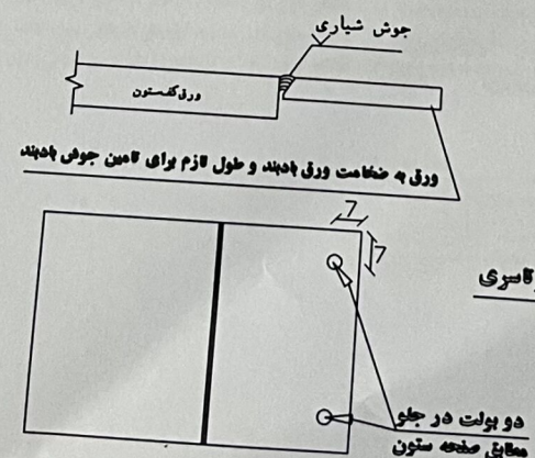
جزئیات اتصال مهاربند 2 UNP120 در اتصال پای ستون در مهاربند ضربدری
