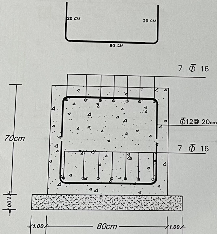
مقطع فنداسیون نواری F-1
