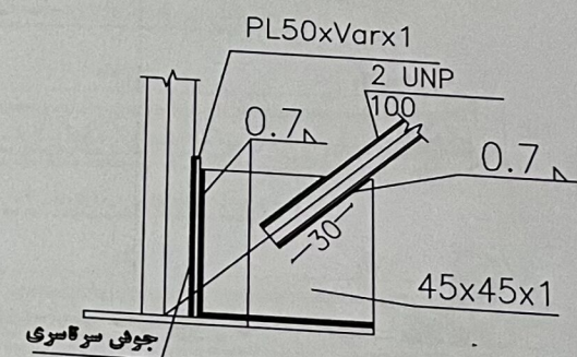
جزئیات اتصال مهاربند 2 UNP100 در اتصال پای ستون در مهاربند ضربدری
