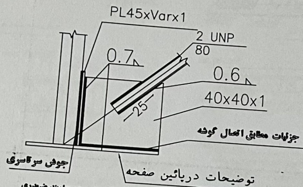
جزئیات اتصال مهاربند 2 UNP80 در اتصال پای ستون در مهاربند ضربدری
