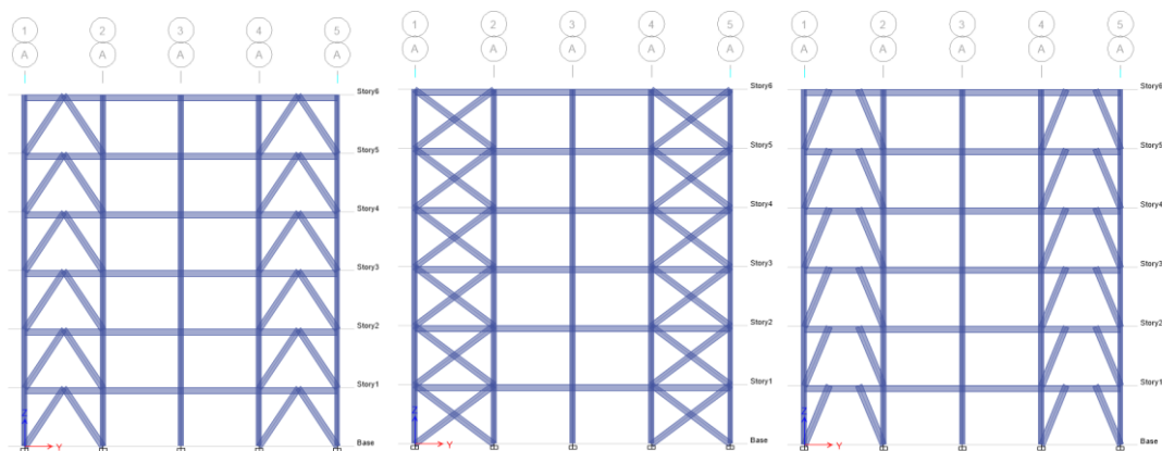
شکل ۲- شکل شماتیک از قاب‌های ۴ دهانه دارای مهاربند X، ۸ و EBF
