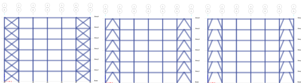
شکل ۳- شکل شماتیک از قاب‌های ۶ دهانه دارای مهاربند X، ۸ و EBF
