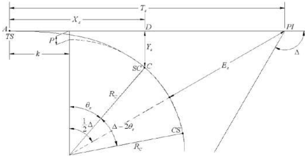
شکل ۴-۱- جزئیات قوس افقی کلوئوئید (اسپیرال).
