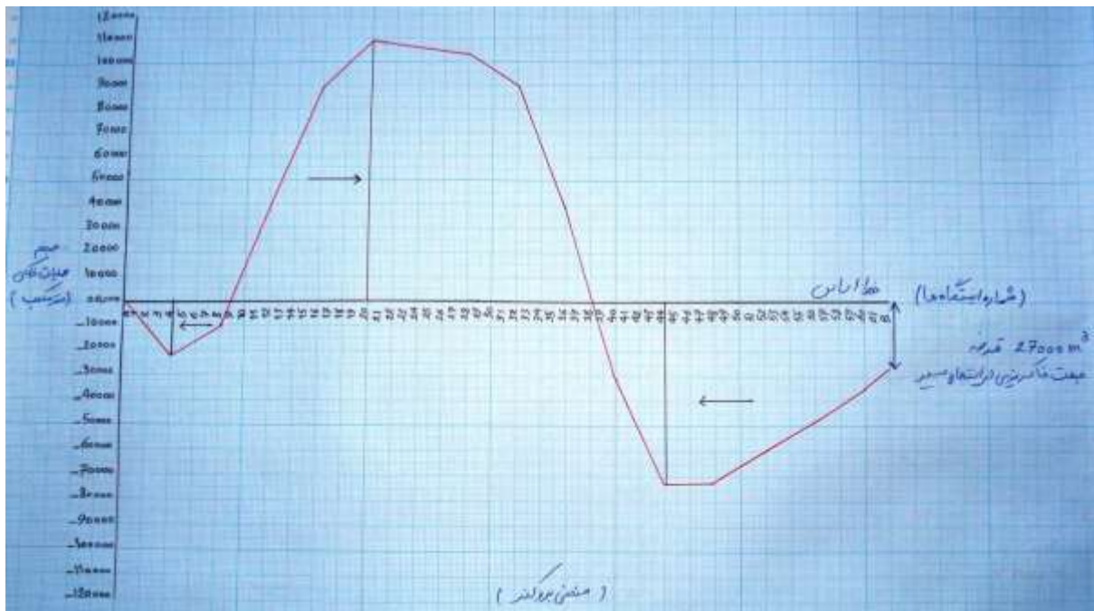
شکل ۱۰-۱- منحنی بروکنر.
