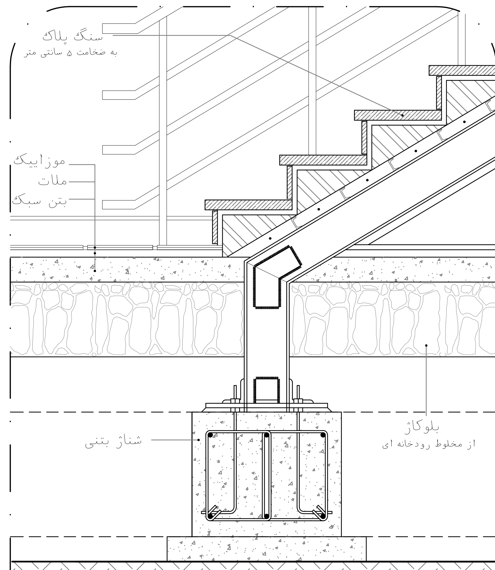
LY.T-10 جزئیات شناژ پله
