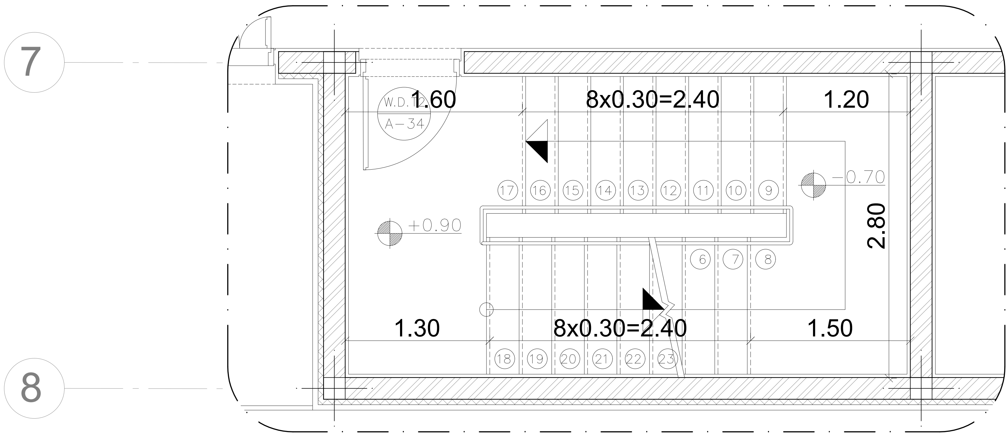
پله طبقه همکف Layout04
