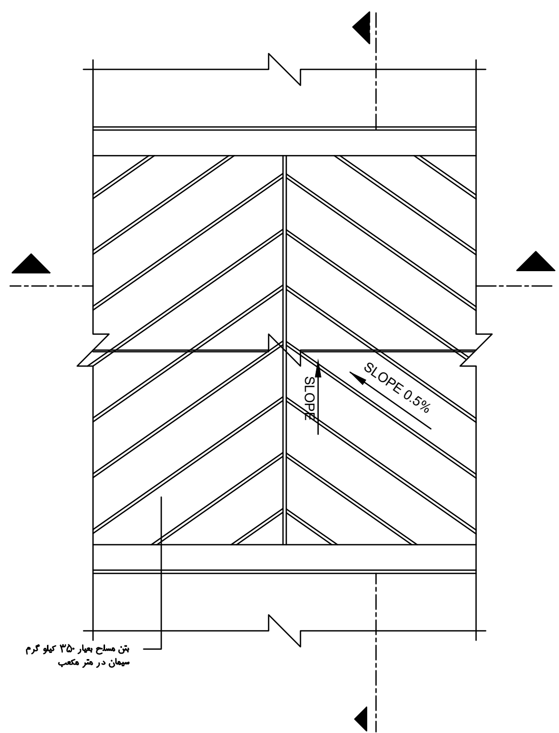
LY.T-13 جزئیات رمپ پارکینگ
