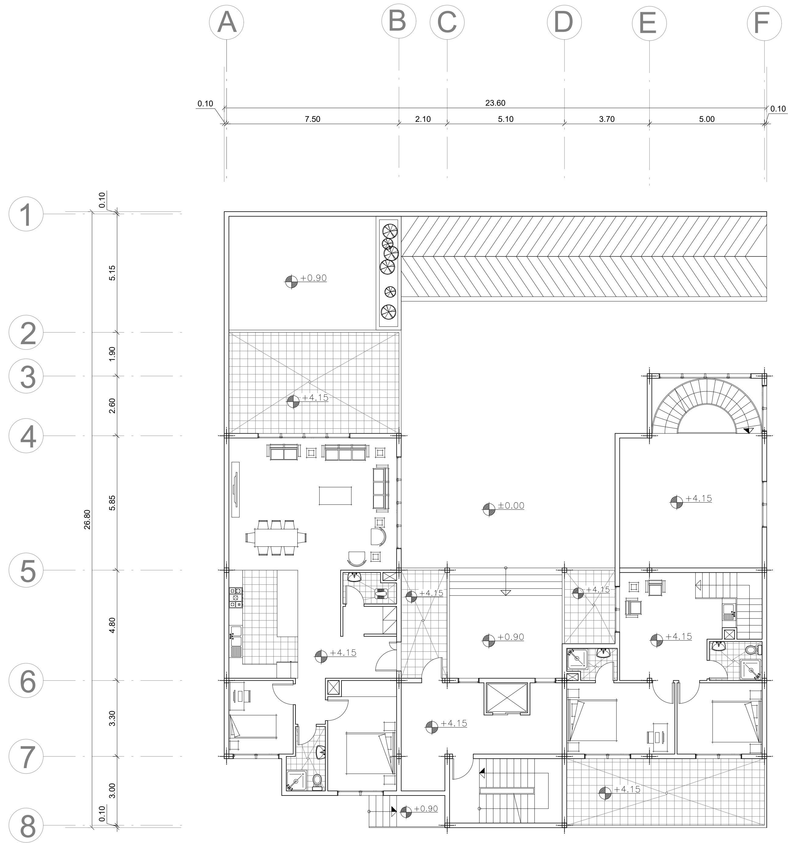
پلان مبلمان طبقه اول
