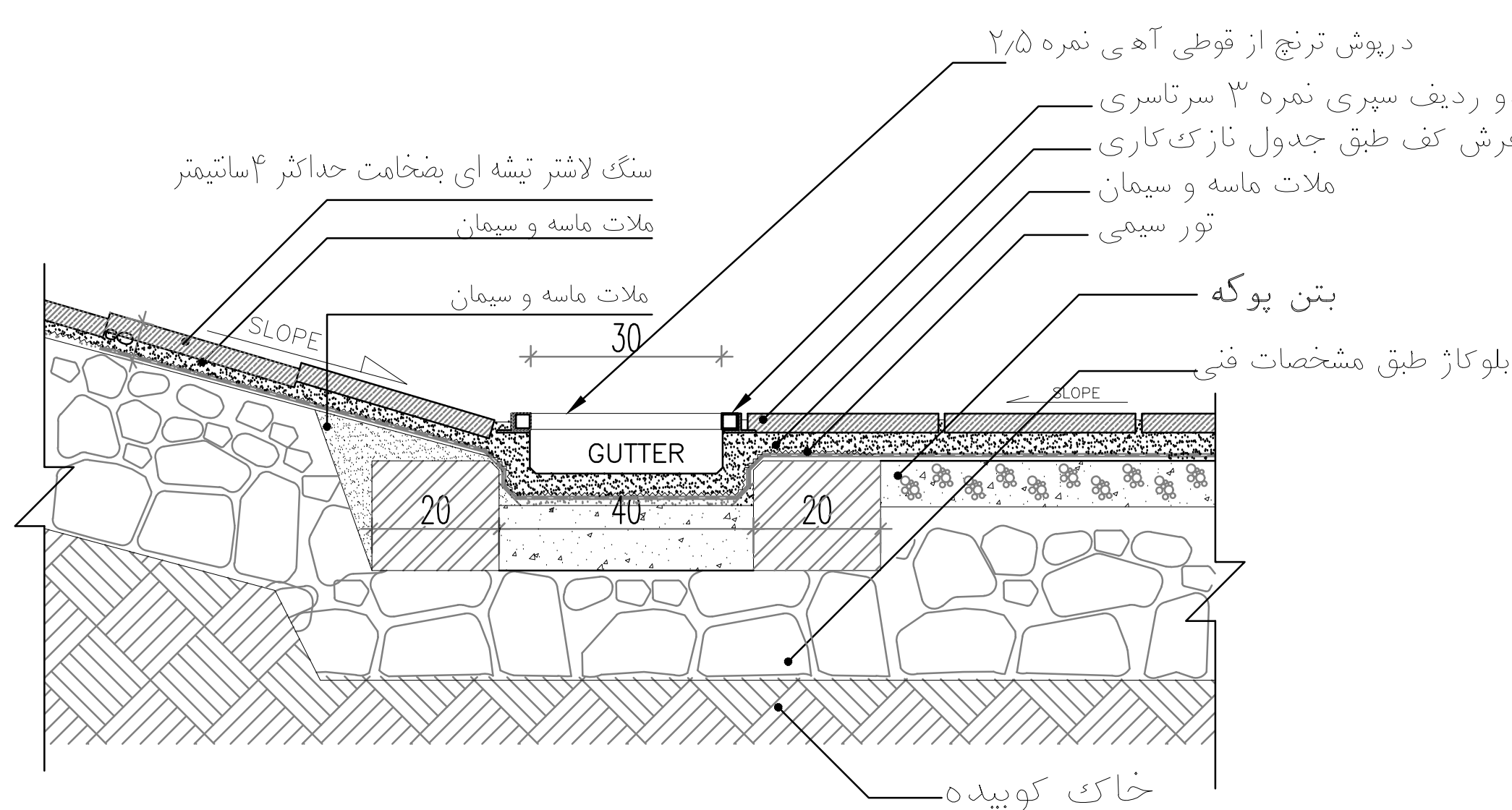
LY.T-13 جزئیات رمپ پارکینگ
