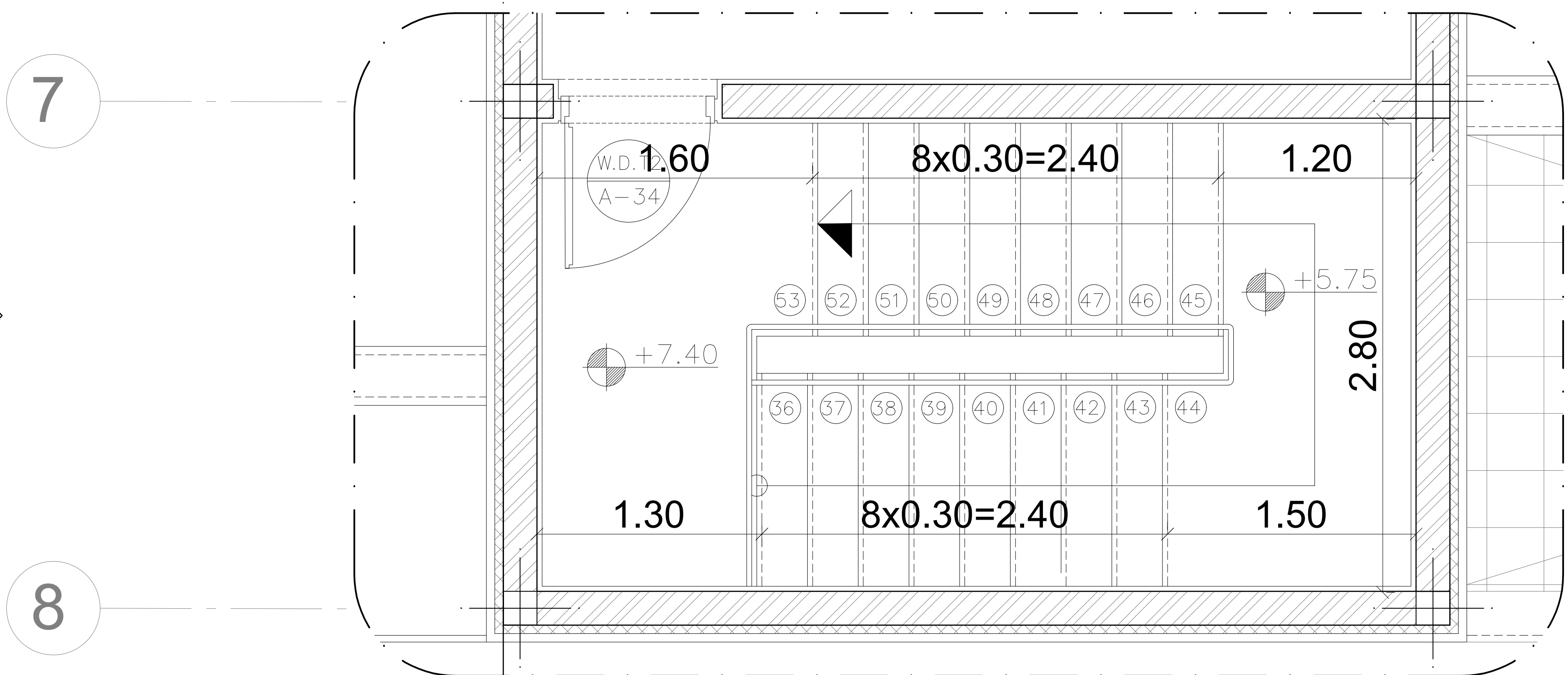
پله از خرپشته
