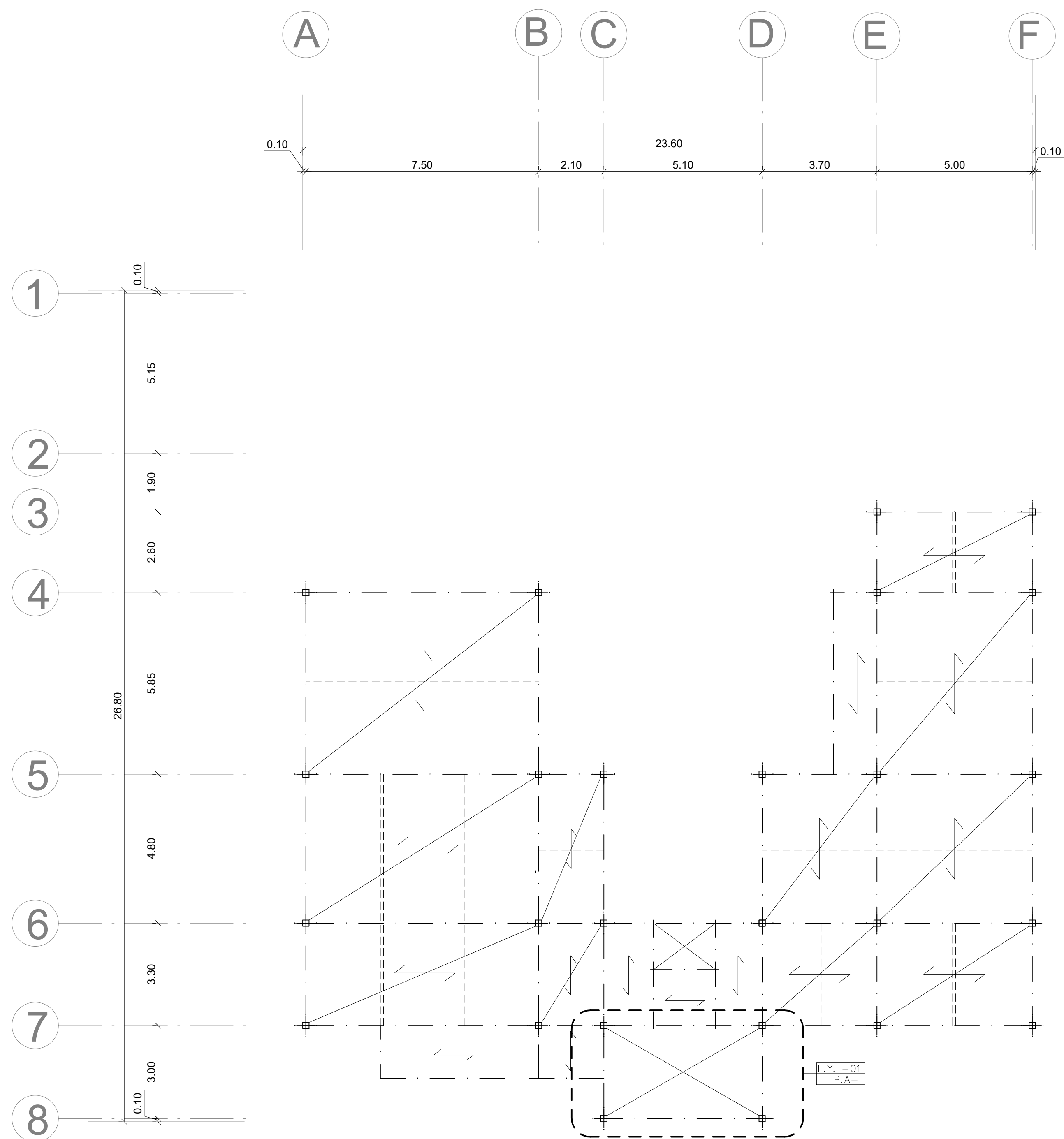
پلان تیرریزی سقف طبقه اول
