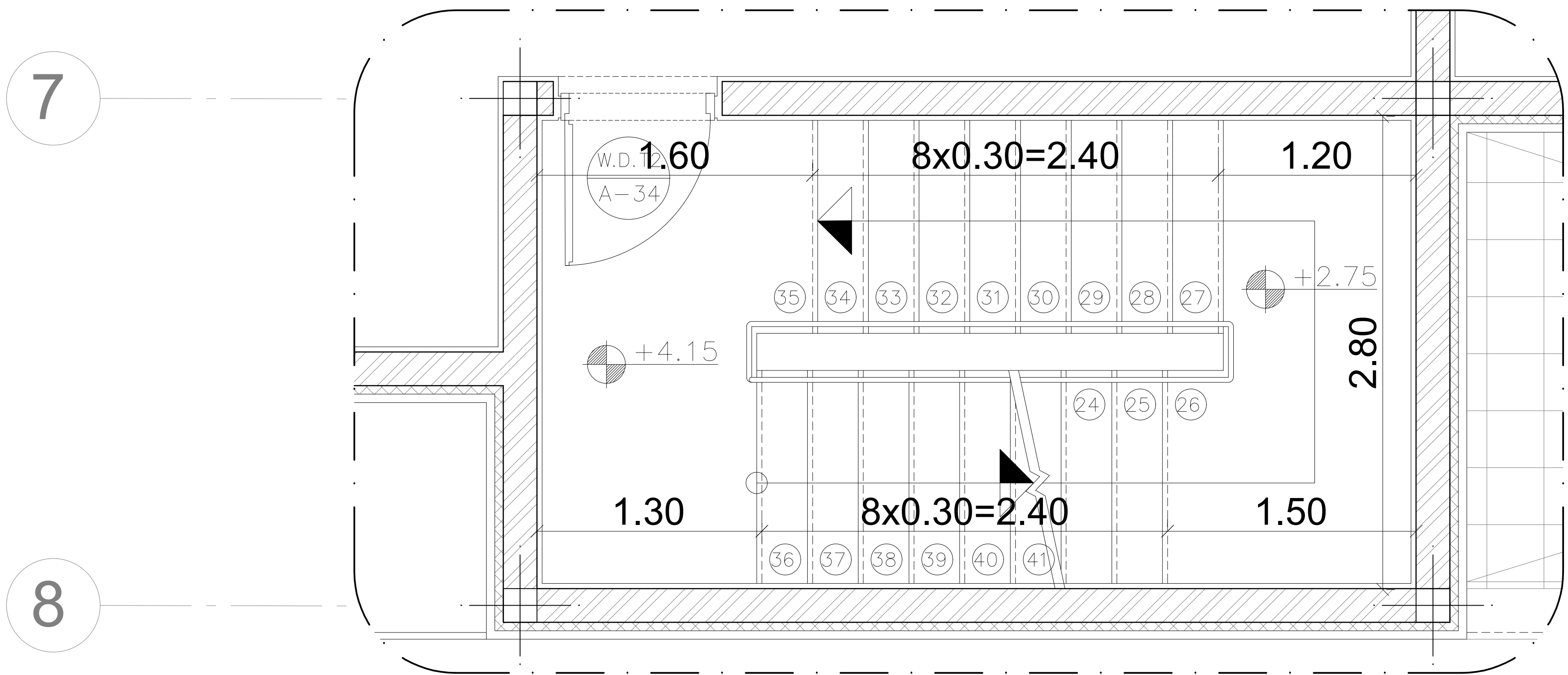
پله طبقه اول Layout05
