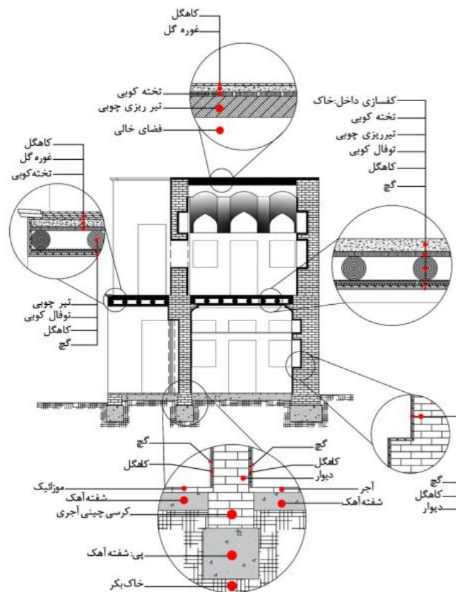
شکل ۴-۱۰- جزئیات بی تا سقف جبهه شمالی بنا (نگارنده)
