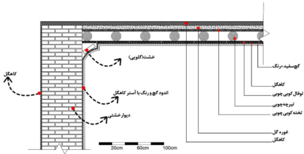
شکل ۴-۱۵- جزئیات اجرایی پوشش تخت در بنا در مقطع عرضی (نگارنده)
